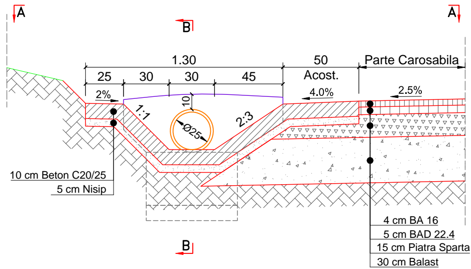
Secțiune Transversala Podet E - E
