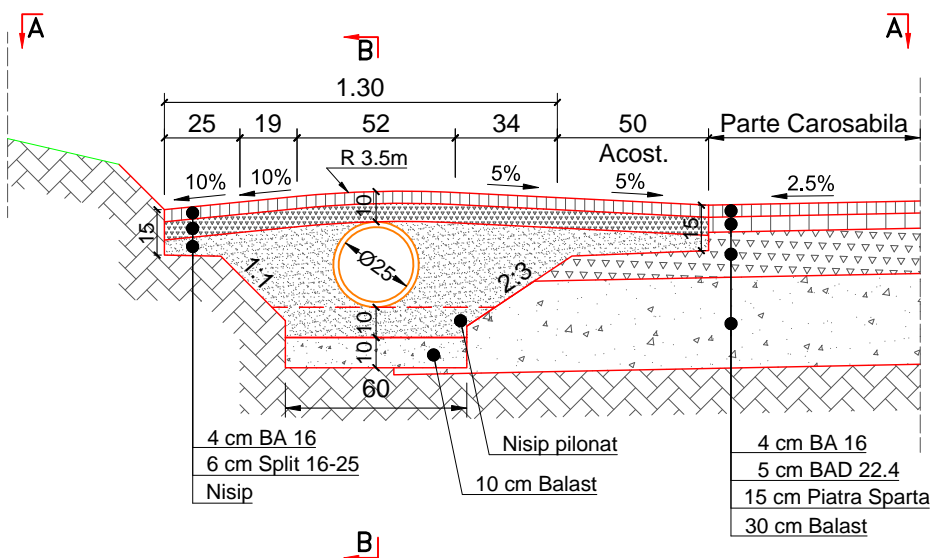
Secțiune Transversala Podet C - C
