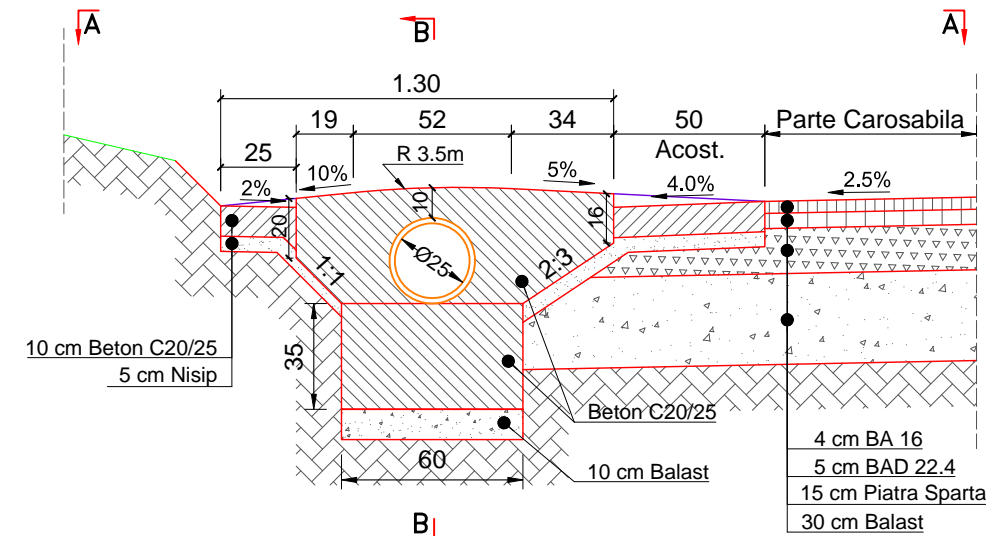
Secțiune Transversala Podet D - D
